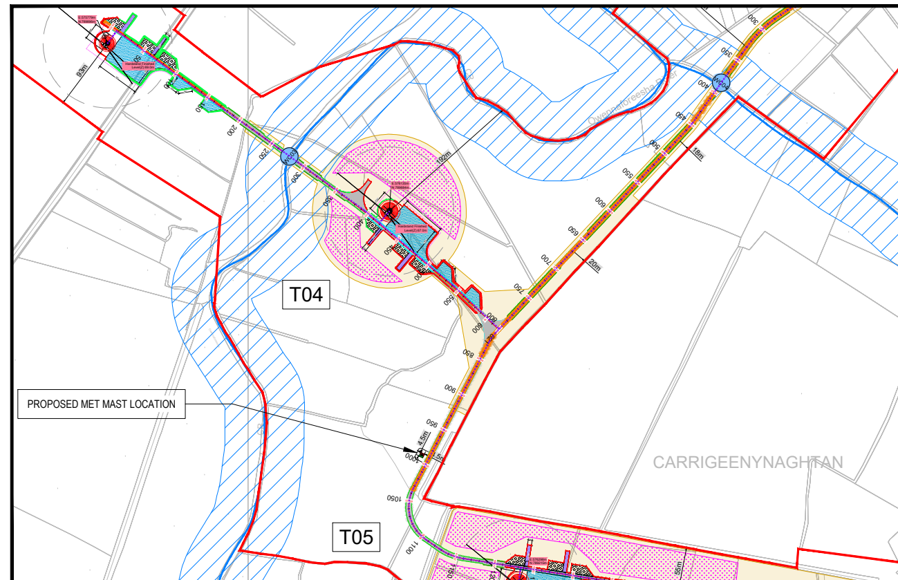
Site Layout Plan Scale: N.T.S (A3)
